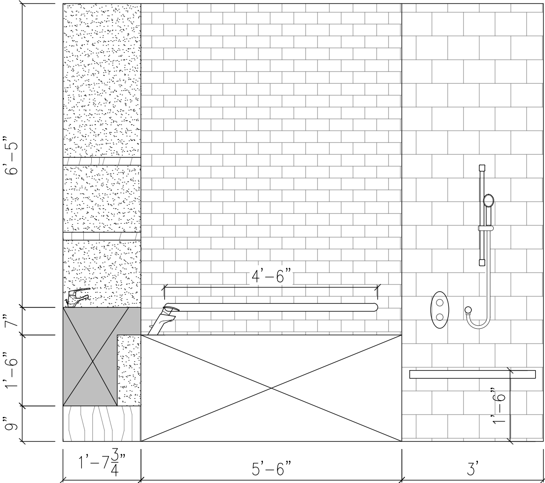
ELEVATION 1
