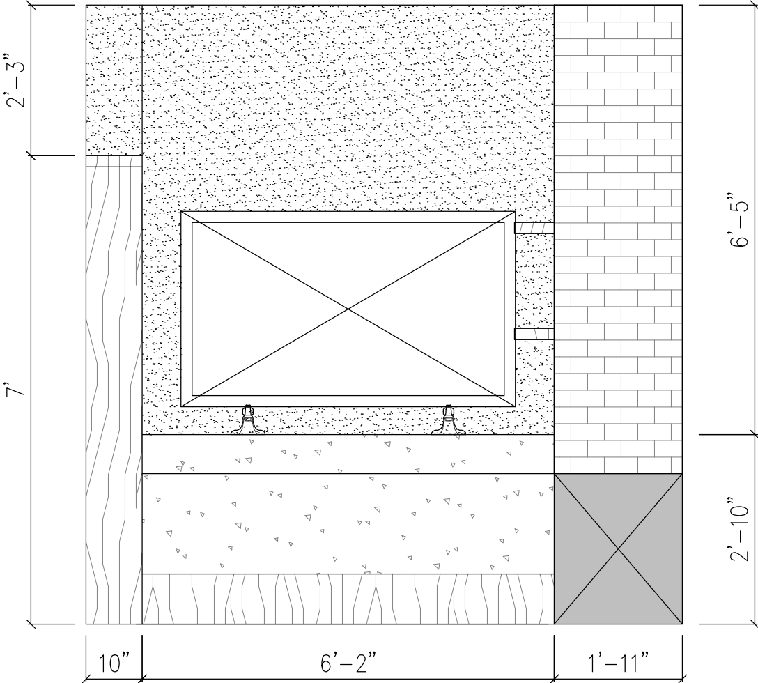
ELEVATION 2
