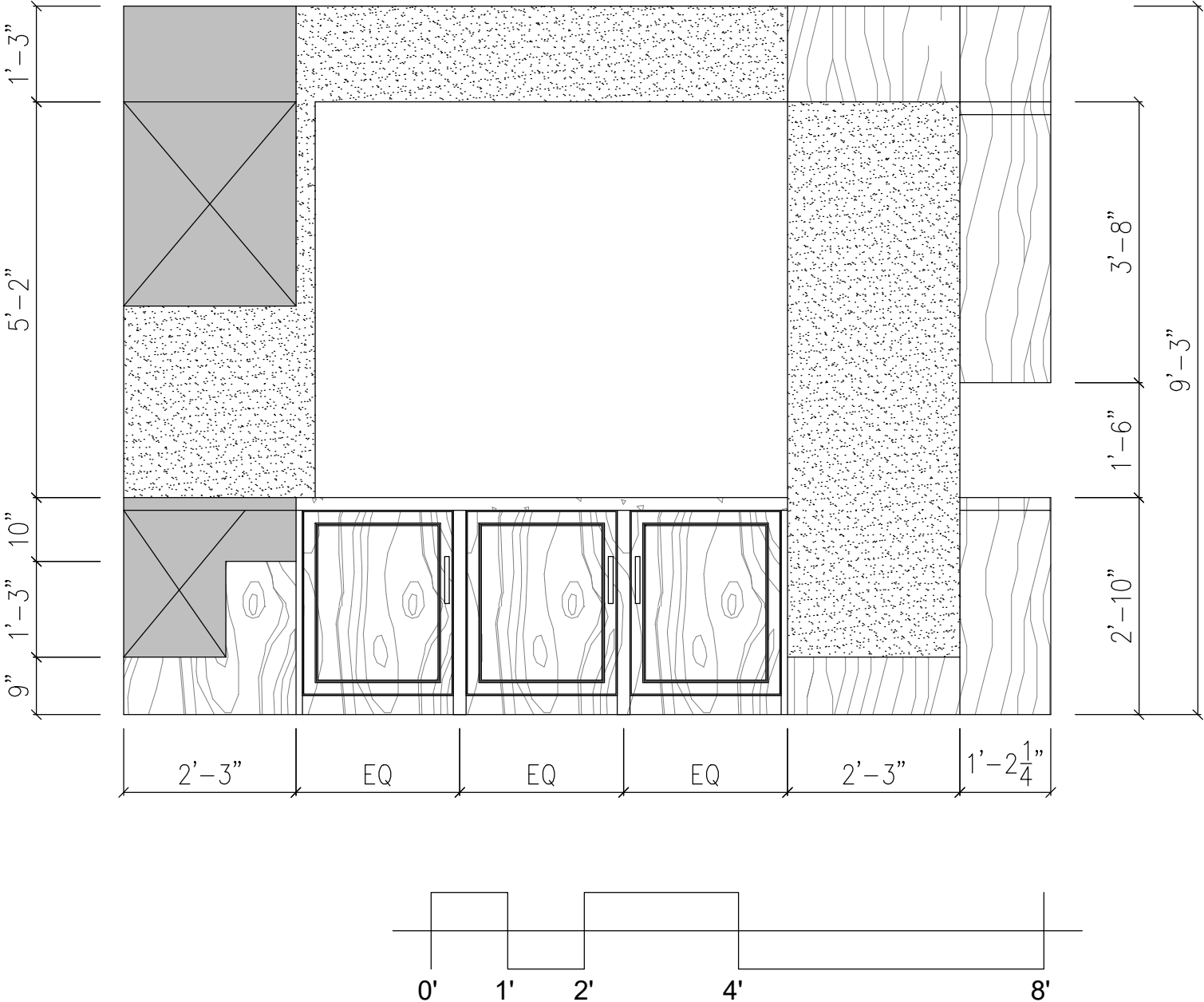
ELEVATION 2
